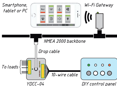
Basis systeem met enkele Circuit Control
