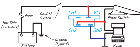
Figuur 2. Handmatig/automatisch met Smart Relay
