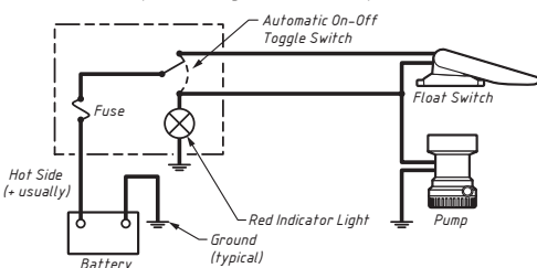
Figuur 1. Schema voor de conventionele methode
